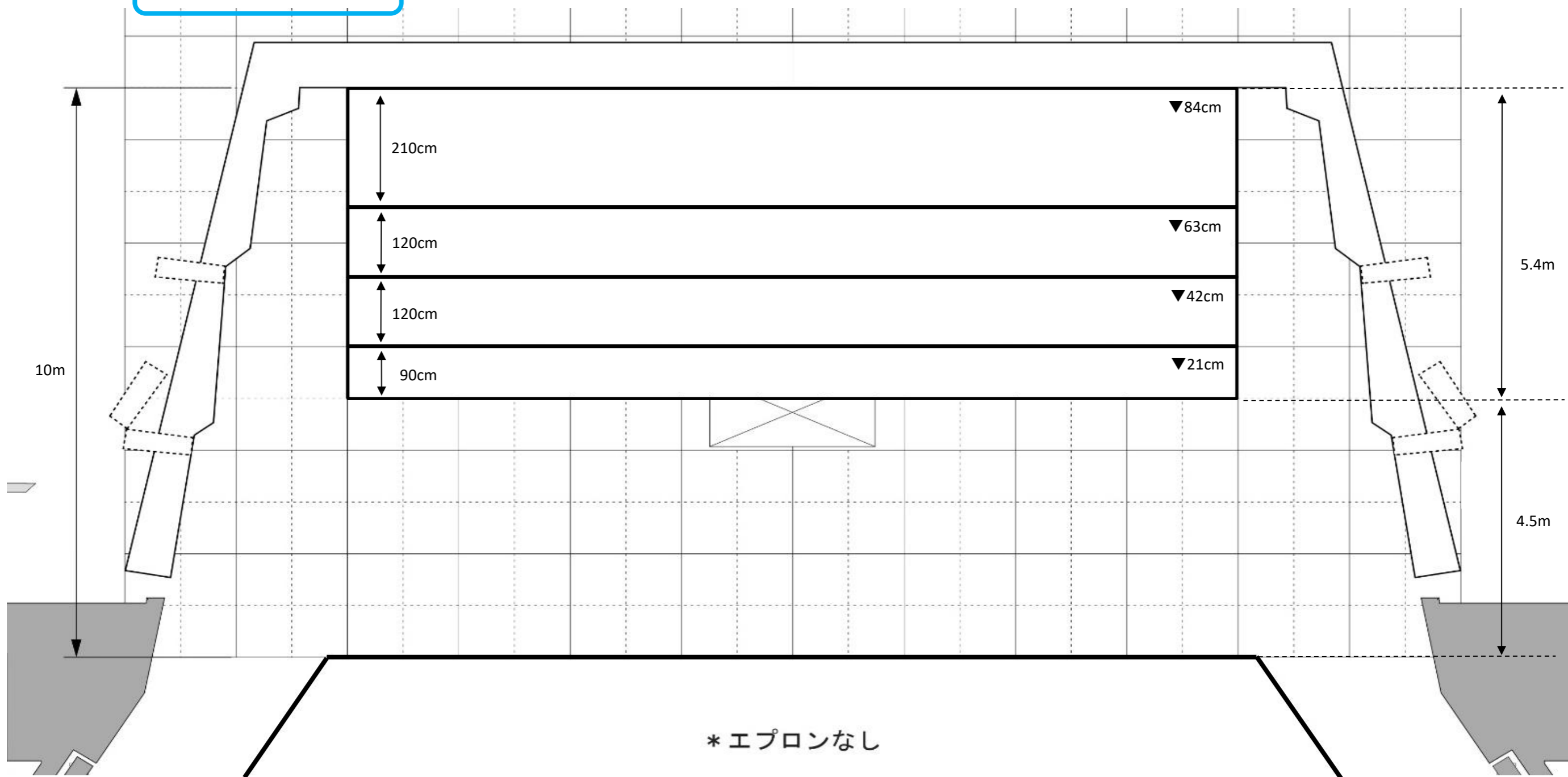
大ホール舞台平面図
